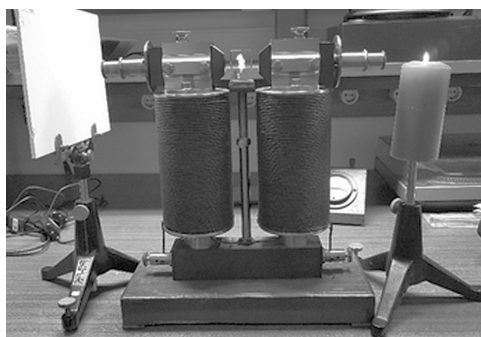
Figura 3: Experiência da Rotação de Faraday – Museu Faraday.
