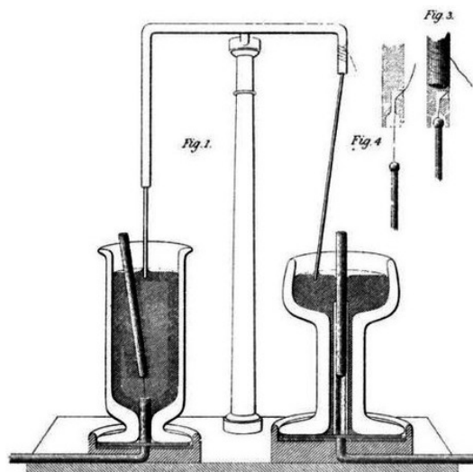
Figura 1: A primeira experiência de Faraday mostrando a transformação de energia eletromagnética em energia mecânica.
