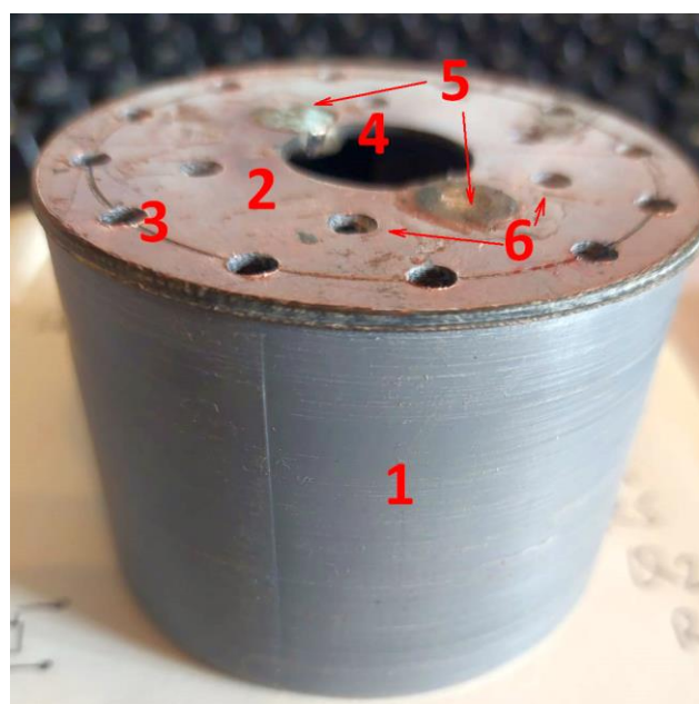
Fig. 13- Interior amovível do cálice.
