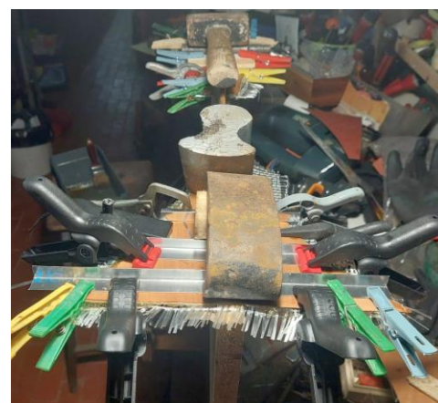
Fig. 16 - Moldagem das lâminas da madeira compósita.
