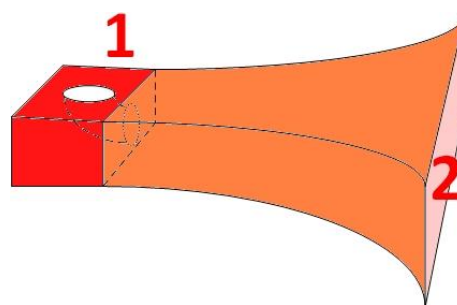
Fig. 14 – Corneta acústica.
