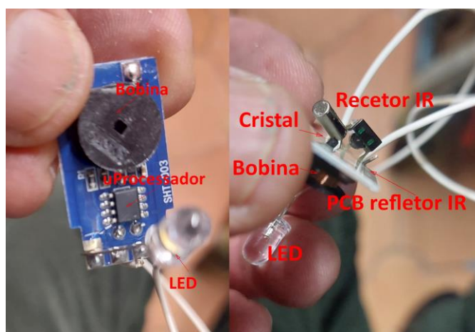
Fig. 5 – Mecanismo da vela grossa.
