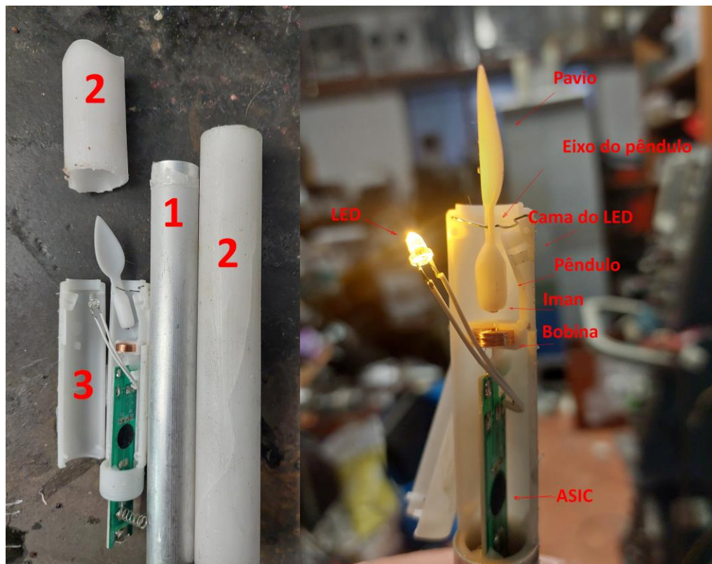
Fig. 4. - Vela fina – 1 – Invólucro de alumínio; 2- invólucro de cera, 3- mecanismo pendular do pavio.
