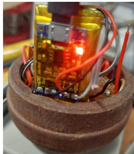
Fig. 10 – Módulo da bateria e respetivos circuitos de proteção e de carregamento.
