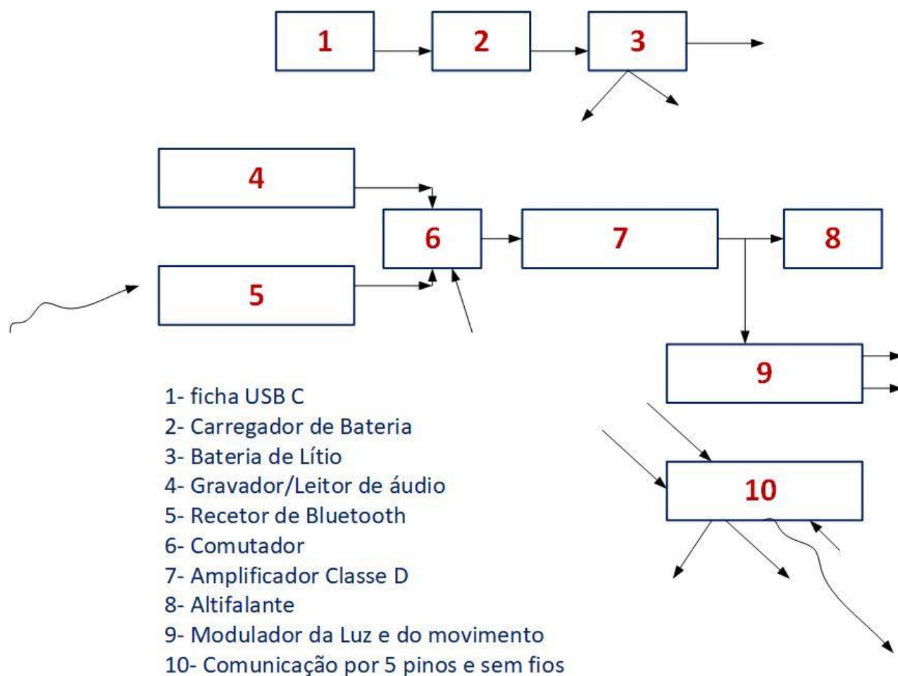
Fig. 1- Arquitetura das velas e do castiçal Faraday.
