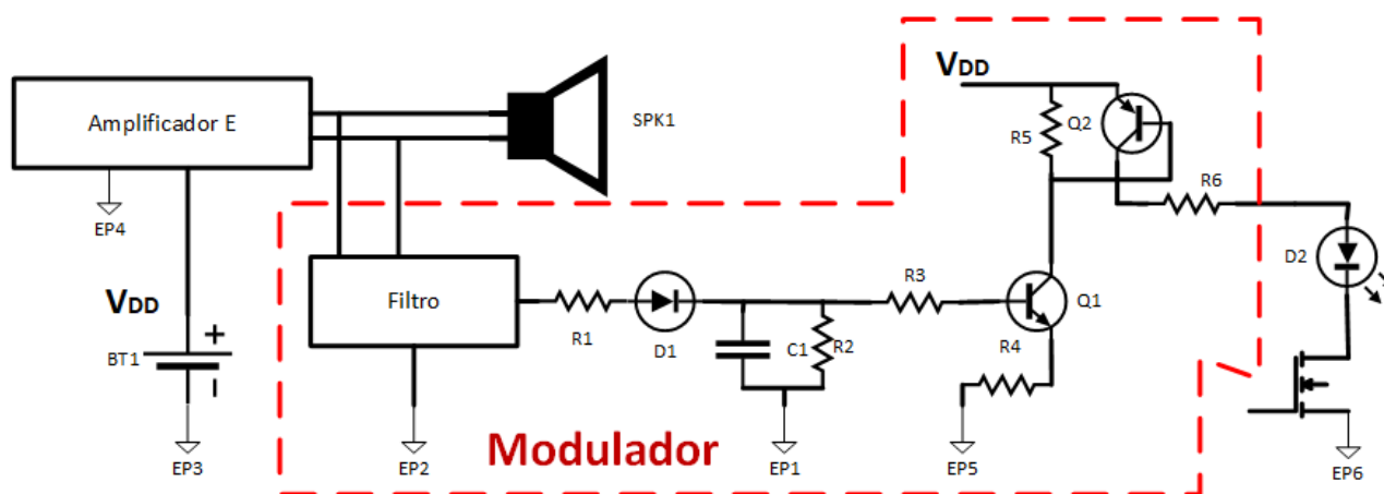
Fig. 11- Representação do circuito de modulação da luz do pavio.
